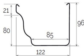
Sezione GRB120
