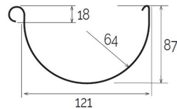
Sezione GR145
