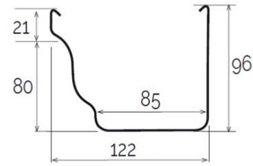
Sezione GRB120
